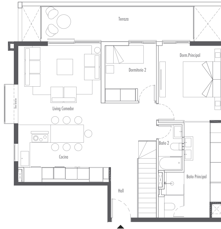
PISO 2
