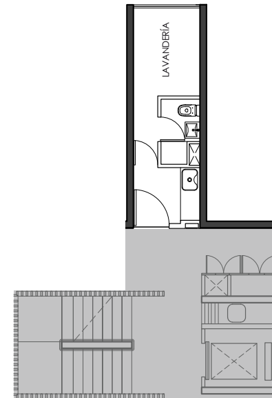
PISO 5
