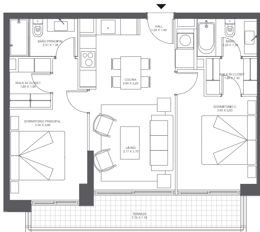
PISO 2
